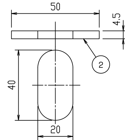
"B"部詳細
