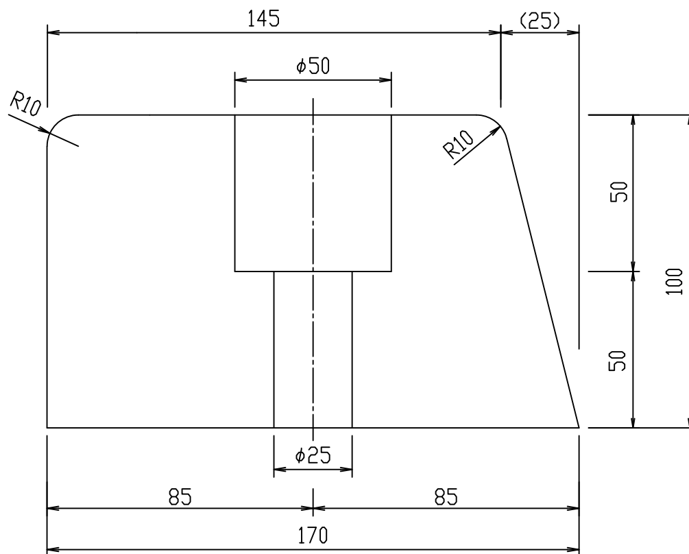
A-A断面
